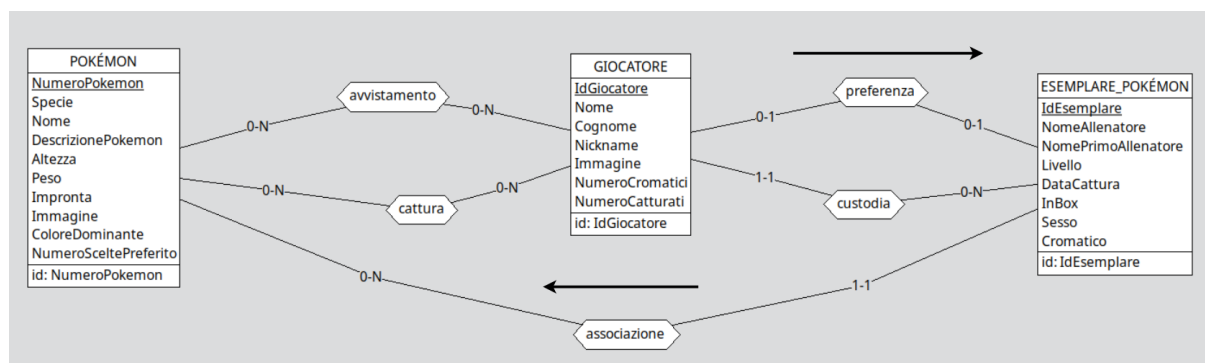
Figura 3.1: Schema di navigazione per cambiare il Pokémon preferito di un giocatore
