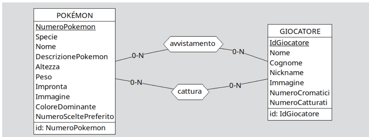
Figura 2.3: Schema ER rappresentante il completamento del Pokédex di un giocatore quando trova e cattura Pokémon per la prima volta
