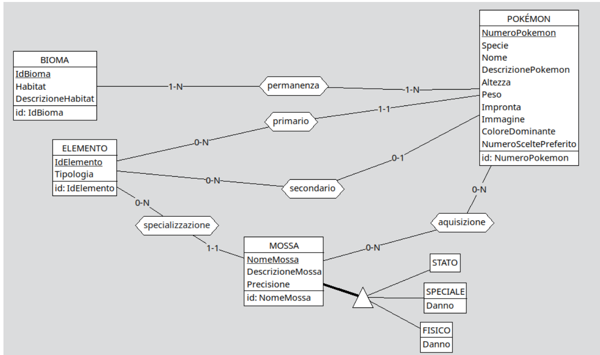
Figura 2.5: Schema ER contenente le entità e relazioni per rappresentare gli ELEMENTI che influiscono su habitat e natura dei Pokémon
