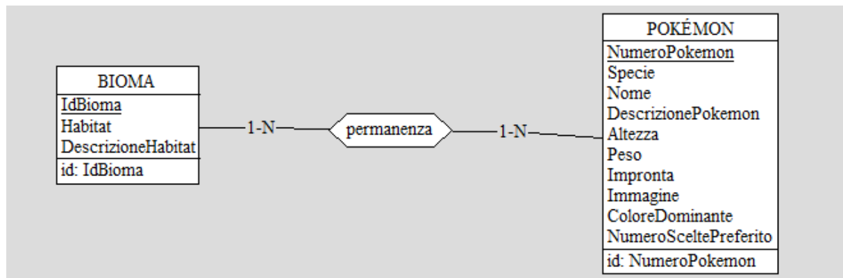
Figura 2.11: Schema ER rappresentante la relazione tra un Pokémon e il bioma a cui appartiene
