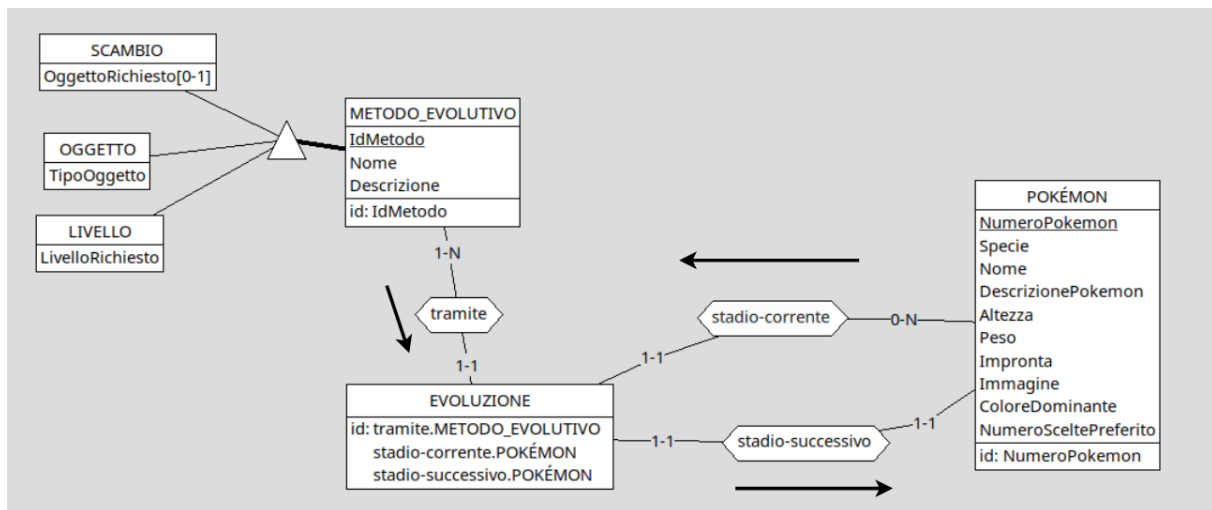
Figura 3.3: Schema di navigazione per visualizzare i Pokémon che si evolvono tramite un certo metodo evolutivo
