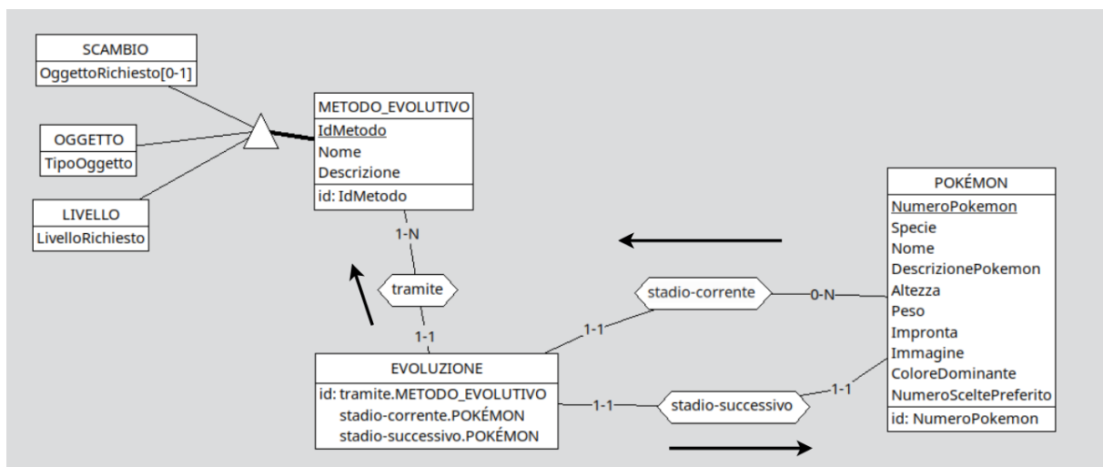
Figura 3.2: Schema di navigazione per visualizzare la linea evolutiva di un Pokémon
