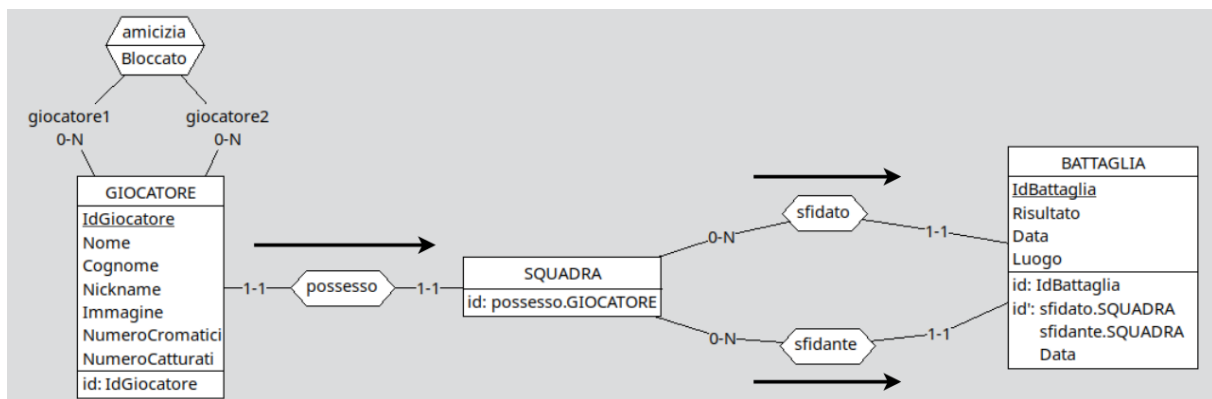
Figura 3.5: Schema di navigazione per visualizzare lo storico delle battaglie dei giocatori
