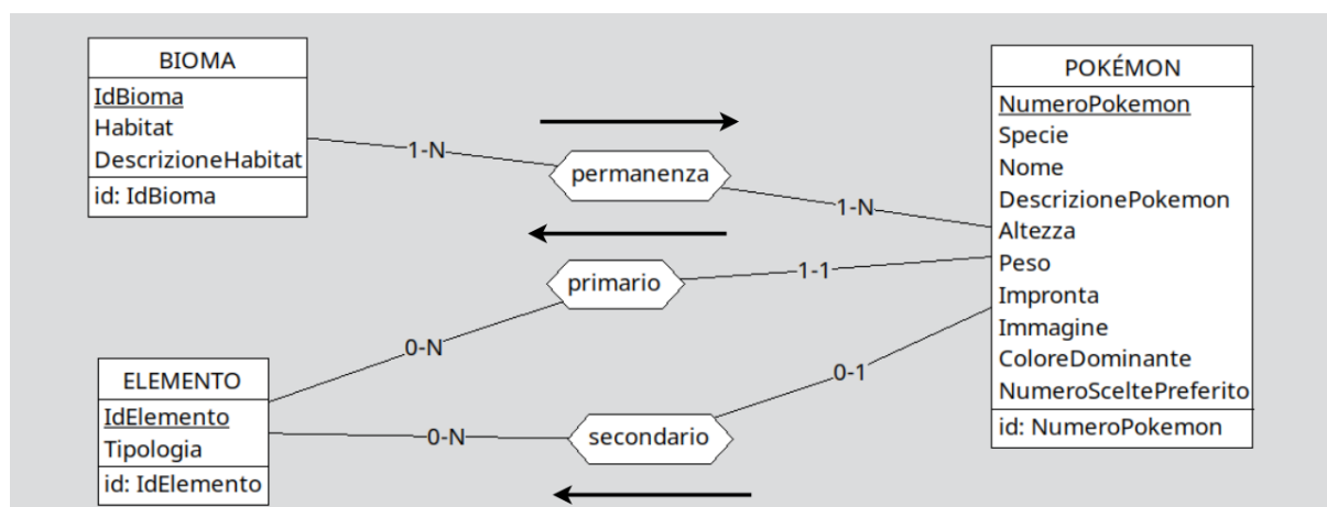
Figura 3.4: Schema di navigazione per visualizzare gli elementi di Pokémon che appartengono allo stesso bioma
