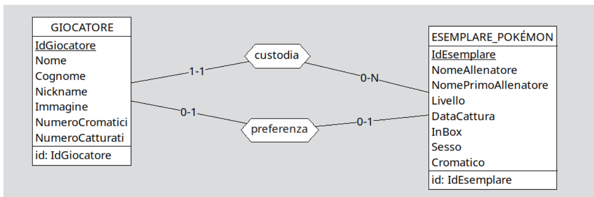
Figura 2.2: Schema ER rappresentante la relazione tra un giocatore e il suo esemplare preferito
