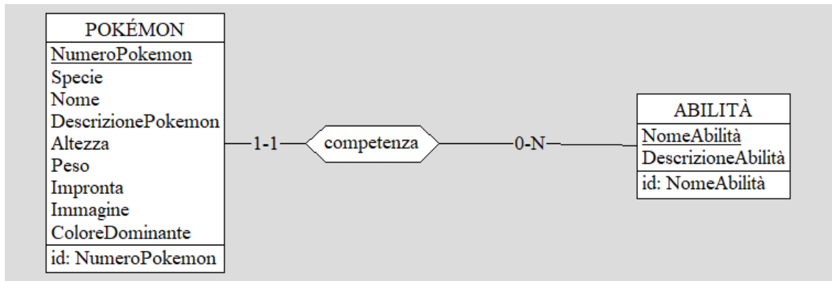
Figura 2.9: Schema ER rappresentante la relazione tra un Pokémon e la sua abilità
