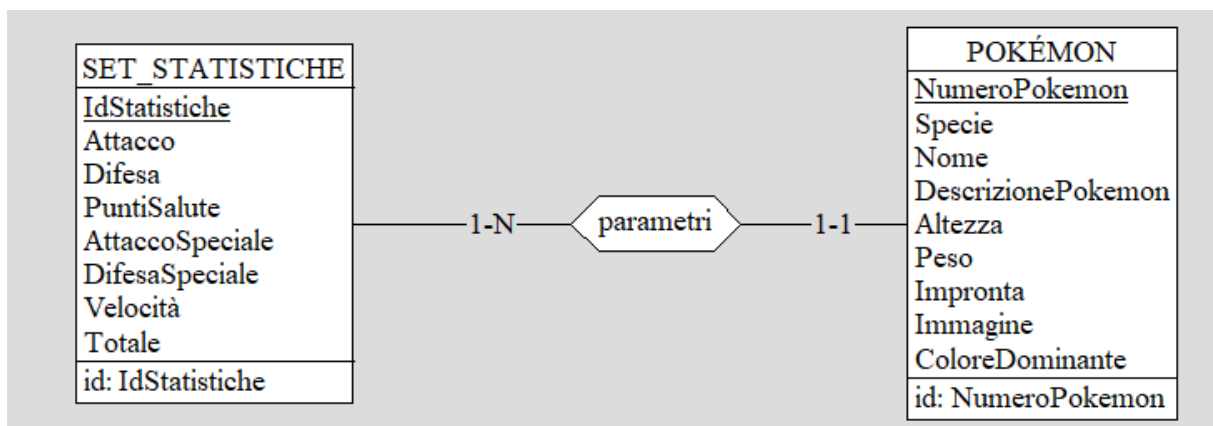
Figura 2.10: Schema ER rappresentante la relazione tra un Pokémon e il suo set di statistiche
